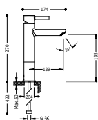
Single lever washbasin mixer with base extension Monocomando lavabo con prolunga inferiore Jednápáková umyvadlová baterie s nástavcem
