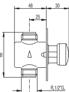
Urinal tap 1/2" G.
