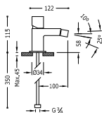
Single lever bidet mixer Monocomando bidet Jednopáková bidetová baterie
