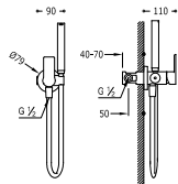
Monocomando ad incasso per bidè WC Supporto a destra o a sinistra, intercambiabile. Flesso satinato.
