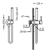
Concealed single lever bidet/toilets Left or right support, interchangeable. Sateen hose. Monocomando ad incasso per bidé WC Supporto a destra o a sinistra, intercambiabile. Flesso satinato. Jednápáková podomítková baterie pro bidet WC Výměnitelný držák zprava či zleva. Sprchová mosazná baterie s omešovacím hrdlem 5 l/m. Systém proti kapání a flexi hadice SATIN
