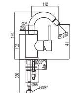
Single lever bidet mixer Monocomando bidet Jednápáková bidetová baterie
