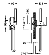
Monocomando ad incasso per bidè WC Supporto a destra o a sinistra, intercambiabile. Flesso satinato. Opzione Cartongesso
