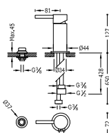
Bidet mixer tap with small shower head Monocomando bidet con doccia Jednopáková bidetová baterie se sprškou
