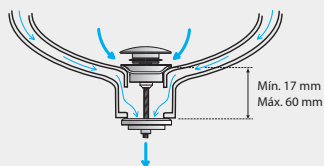
Counter top with overflow drain Piano con troppopieno Deska s přepadem
