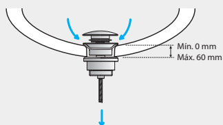
Counter top without overflow drain Piano senza troppopieno Deska bez přepadu
