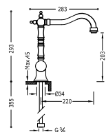
Single lever single hole sink mixer Monocomandoavello verticale Jednopáková dřezová kuchyňská baterie
