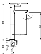
Single lever washbasin mixer with base extension Monocomando lavabo con prolunga inferiore Jednápáková umyvadlová baterie s nástavcem
