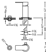
Bidet mixer tap with small shower head Monocomando bidet con doccetta Jednápáková bidetová baterie se sprškou
