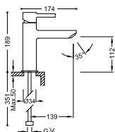
Single lever washbasin mixer Monocomando lavabo Jednápáková umyvadlová baterie
