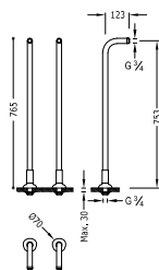
Water intake at floor of bath 2 units Prese d'acqua a terra per vasca da bagno 2 unità Vodovodní přípojky na okraj vany 2 kusy
