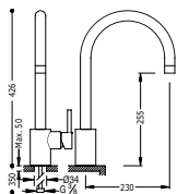
Single lever single hole sink mixer Monocomandoavello verticale Jednopáková dřezová kuchyňská baterie
