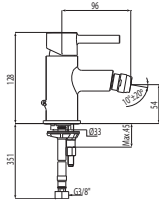
Single lever bidet mixer Monocomando bidet Jednápáková bidetová baterie
