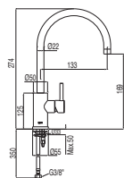
Single lever washbasin mixer Monocomando lavabo Jednápáková umyvadlová baterie
