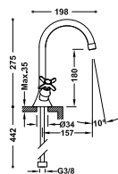
Single hole wash-basin mixer Monoblocco lavabo Dvoupáková umyvadlová baterie
