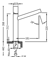
Single lever washbasin mixer long spout Monocomando lavabo canna lunga Jednopáková umyvadlová baterie dlouhé ramínko
