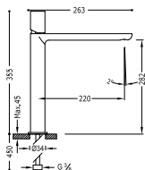
Single lever washbasin mixer Monocomando lavabo Jednárková umyvadlová baterie
