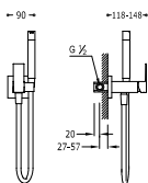
Concealed single lever bidet/toilets Left or right support, interchangeable. Sateen hose. Monocomando ad incasso per bidé WC Supporto a destra o a sinistra, intercambiabile. Flesso satinato.
