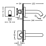
Wall spout Canna parete Nástěnné ramínko
