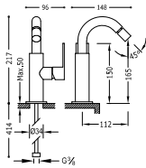
Single lever bidet mixer Monocomando bidet Jednápáková bidetová baterie
