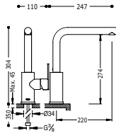
Single lever single hole sink mixer Monocomando lavello verticale Jednopáková dřezová kuchyňská baterie
