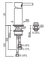
Bidet mixer tap with small shower Monocomando bidet con doccetta Jednápáková bidetová baterie se sprškou
