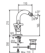
Single hole bidet mixer Monoblocco bidet Dvoupáková bidetová baterie
