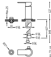
Bidet mixer tap with small shower head Monocomando bidet con doccia Jednopáková bidetová baterie se sprškou
