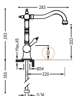
Single hole sink mixer FOLDING Monocomandoavello verticale ABBATTIBILE Jednopáková dřezová kuchyňská baterie SKLOPNÁ
