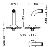
Shower-bath elbow adaptor 2 units with silencer Gomito adattatore bagno-doccia 2 unità con silenziatore Rohový ventil vana-sprcha 2 kusy s tlumičem
