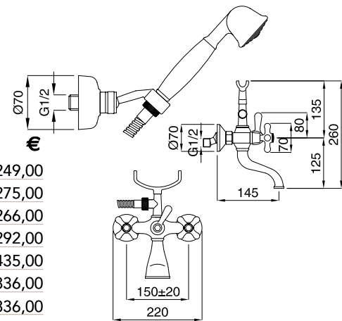
Gruppo vasca esterno con doccia duplex External bath mixer with duplex shower
