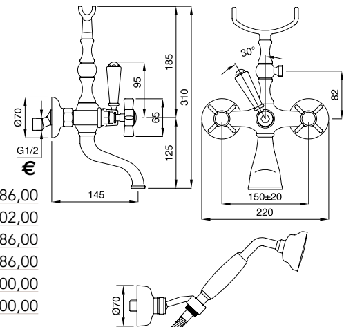
Gruppo vasca esterno con doccia duplex External bath mixer with duplex shower
